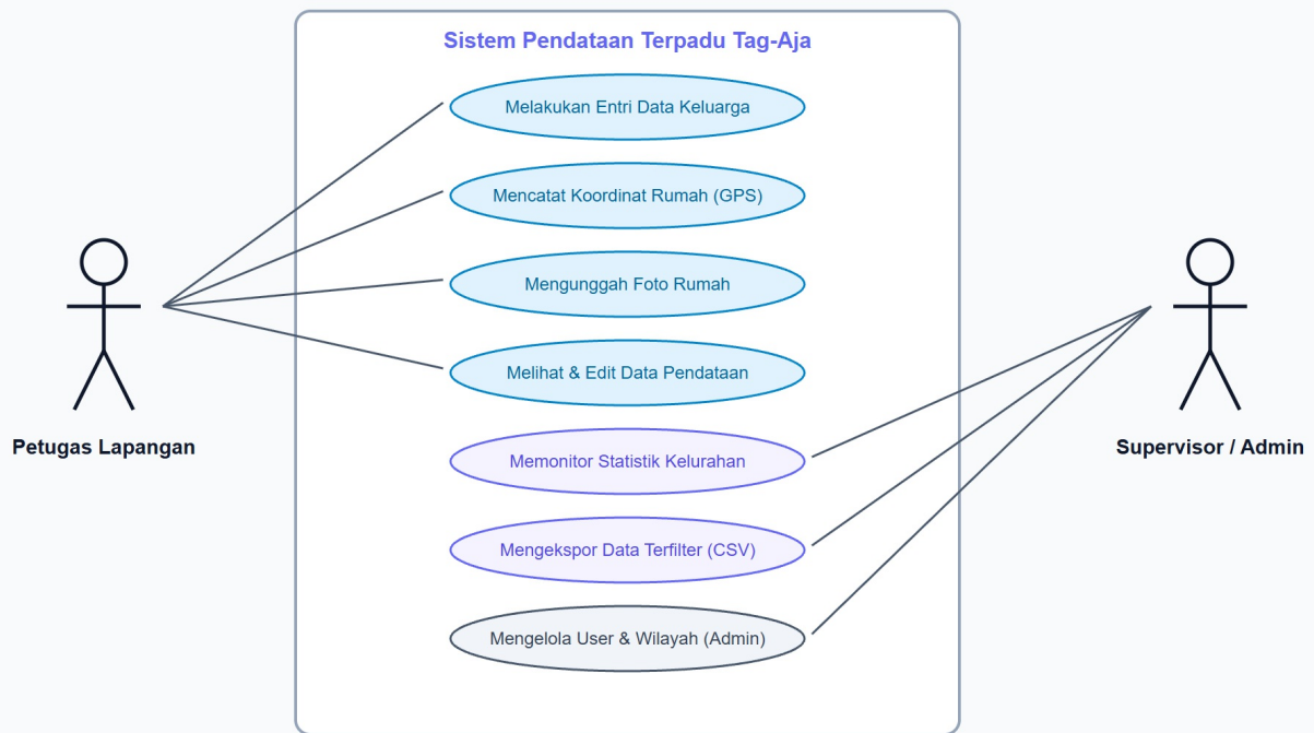
Gambar 3. Diagram Use Case Aplikasi Tag-Aja
