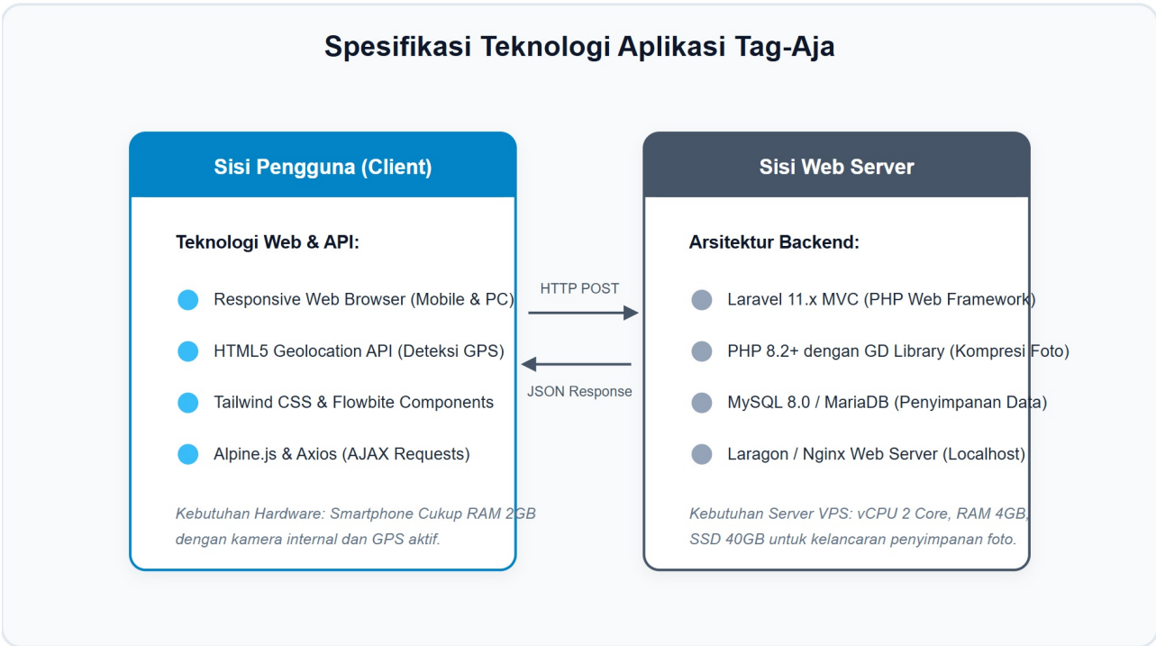
Gambar 2. Spesifikasi Teknologi Aplikasi Tag-Aja
